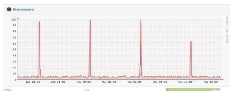
Gambar 1. Grafik Processor
